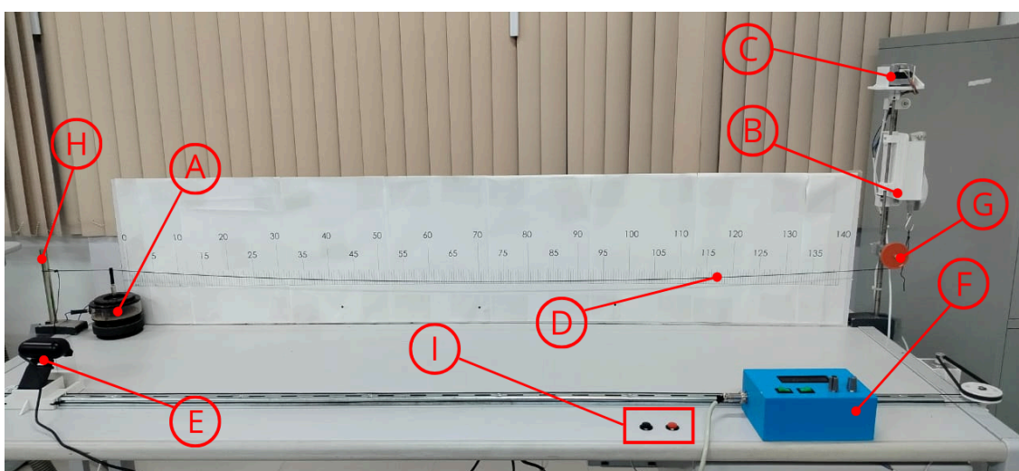
Figura 3: Aparato Híbrido para o Estudo de Ondas Estacionárias.
